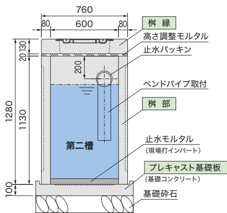
槽内断面図
