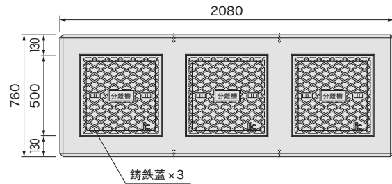
平面断面図
