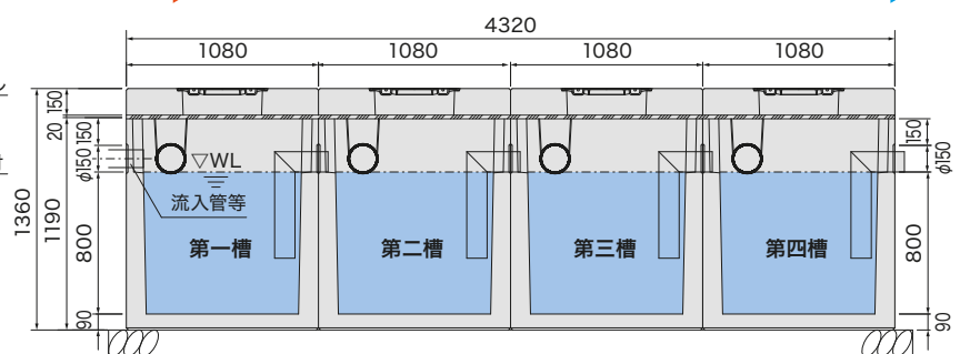
側面断面図
