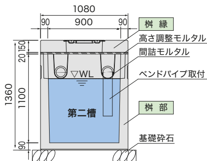
槽内断面図
