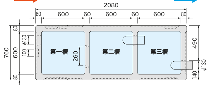
平面断面図
