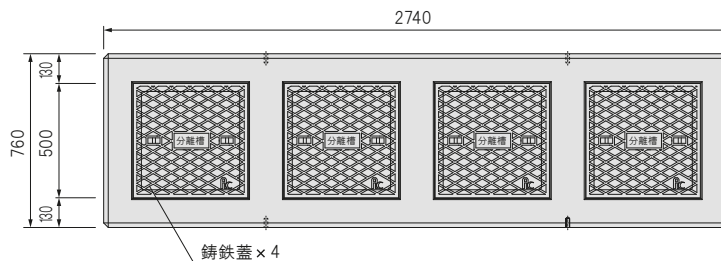
平面断面図
