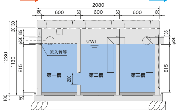
側面断面図
