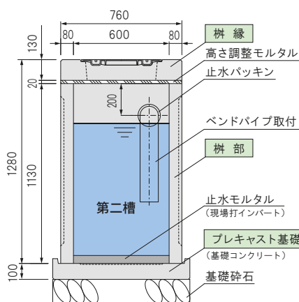
槽内断面図
