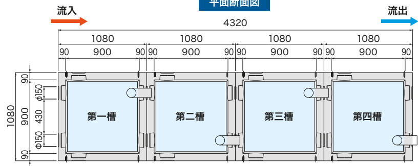
平面断面図
